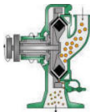
Лопастные мельницы
