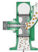
Ударные мельницы
