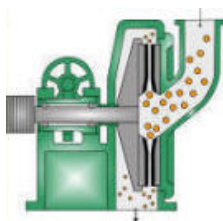
Дисковые мельницы
